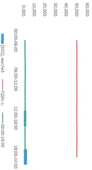
SO 2 , мкг/м 3
