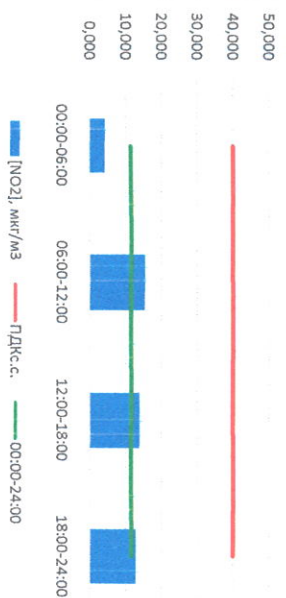
NO 2 , мкг/м 3
